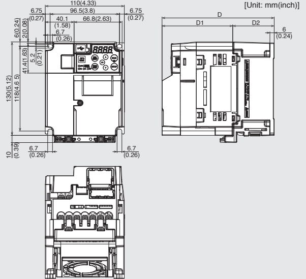
Type FRN0002E3E-4G, FRN0004E3E-4G
