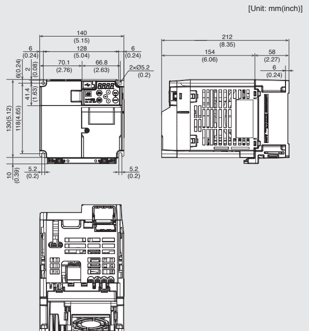
Type FRN0006E3E-4G, FRN0007E3E-4G, FRN00012E3E-4G, FRN0008E3E-7G, FRN0011E3E-7G
